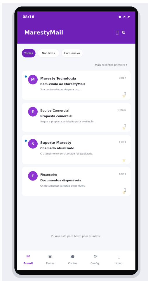
Figura 5 - Filtros “Todas”, “Nao lidas”, “Com anexo” e ordenação da lista.
